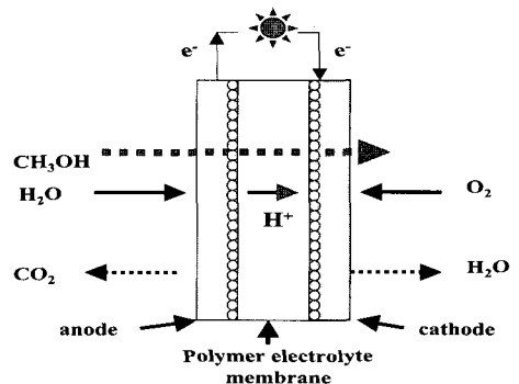
[그림 2] DMFC의 구조 및 원리
