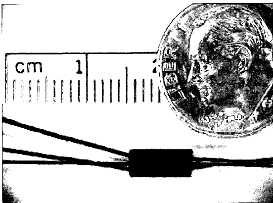
[그림 5] 초소형 개질기 시스템 (100 mWe) (기화기+개질기+연소기)
