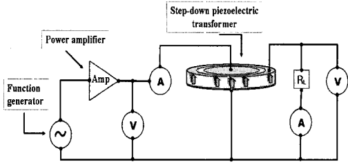
그림 2. 압전변압기 특성측정회로 블록 다이어그램. Fig. 2. Block diagram of piezoelectric transformer driving circuit.
