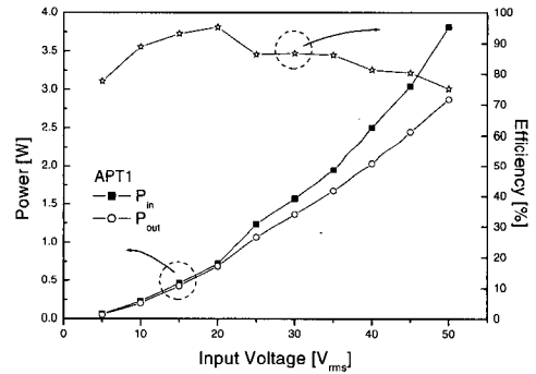
그림 11. 입력력 파워와 효율.
