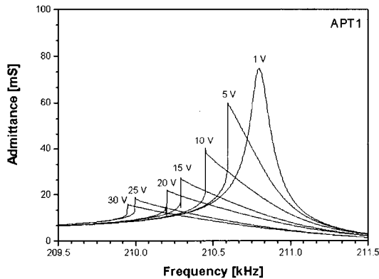
그림 5. 압전 변압기의 어드미턴스 커브.
