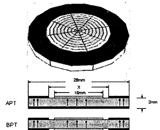
그림 1. 디스크형 압전변압기.
