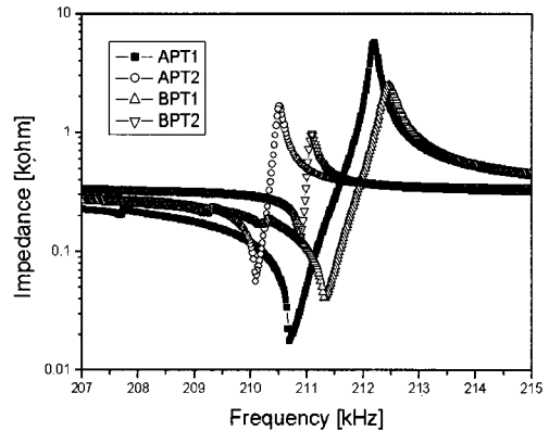
그림 3. 압전 변압기의 임피던스 커브. Fig. 3. Impedance curve of piezoelectric transformer with no load resistance.
