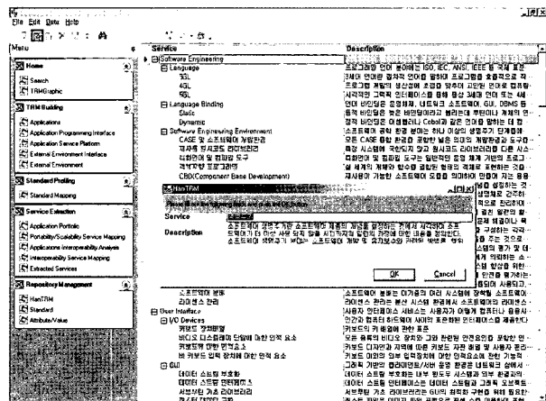
(그림 4) 기술참조서비스 등록
