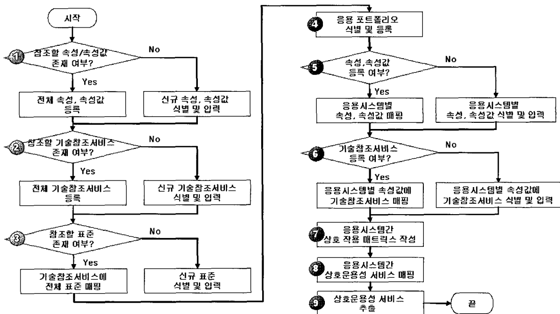
(그림 1) 상호운용성 서비스 추출 알고리즘
