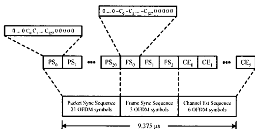
그림 4. MB-OFDM UWB 시스템의 동기화 및 채널 추정을 위한 PLCP 프리앰블 구조
