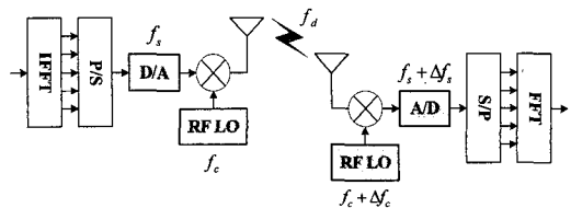
그림 1. 일반적인 OFDM 시스템 송신단에서 반송파 및 샘플링 주파수 오프셋의 발생 위치.
