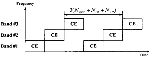
그림 6. MB-OFDM UWB 시스템에서 주파수 도약을 통한 CE 시퀀스 전송의 예(Piconet #1).
