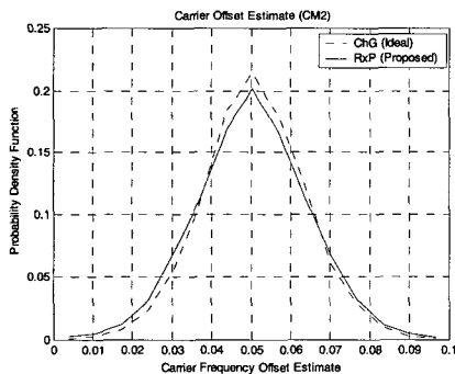
그림 10. 추정 기법에 따른 반송파 주파수 오프셋 추정의 PDF 성능(CM2, Piconet #1, SNR = 15 dB, \epsilon_s = 200 ppm, \epsilon_c = 0.05 ).
