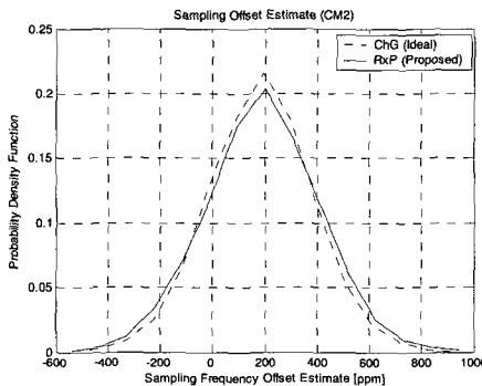
그림 9. 추정 기법에 따른 샘플링 주파수 오프셋 추정의 PDF 성능(CM2, Piconet #1, SNR = 15 dB, \epsilon_s = 200 ppm, \epsilon_c = 0.05 ).
