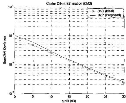
그림 8. 추정 기법과 SNR에 따른 반송파 주파수 오프셋 추정의 표준편차 성능 (CM2, Piconet #1, \epsilon_s = 200 ppm, \epsilon_c = 0.05 ).
