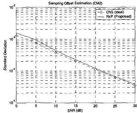
그림 7. 추정 기법과 SNR에 따른 샘플링 주파수 오프셋 추정의 표준편차 성능 (CM2, Piconet #1, \epsilon_s = 200 ppm, \epsilon_c = 0.05 ).
