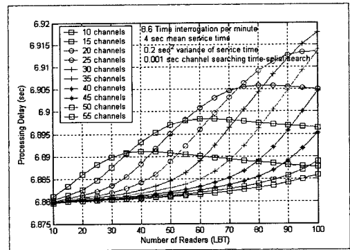
그림 2. 주파수 채널 용량별 최대 처리 트래픽 밀도 및 최대 수용 리더 수
