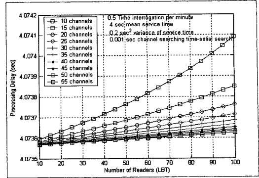
그림 1. 주파수 채널 용량 및 리더 수에 따른 트래픽 처리시간
