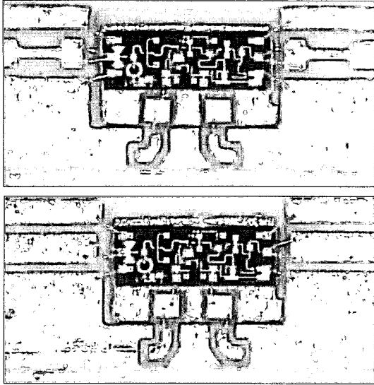
(a) 본드 와이어 매칭된 LNA 회로(위쪽)와 본드 와이어 매칭 안된 LNA 회로(아래쪽) (a) LNA circuit with matched bond-wire(on the up side) and with no matched bond-wire(on the down side)
