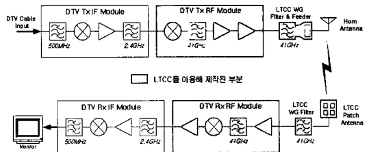
그림 7. DTV 전송 시험 구성도 Fig. 7. DTV transmission test diagram.
