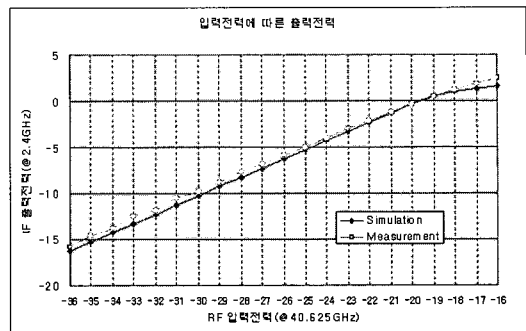
그림 6. LTCC 수신기 모듈의 측정 결과 Fig. 6. Simulated and measured results of receiver module.
