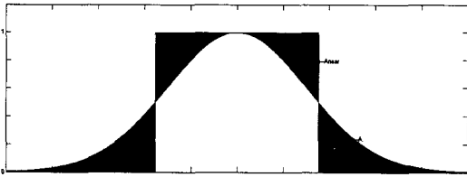
그림 1. 퍼지집합의 엔트로피
