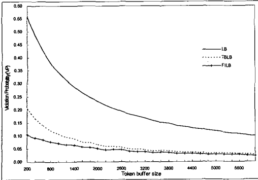
그림 2. 토큰 버퍼 크기에 대한 LB, TBLB 그리고 FILB의 셀 위반 확률
