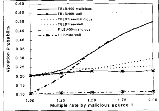
그림 3. 계약 위반 소스에 대한 각 연결이 셀 위반 확률
