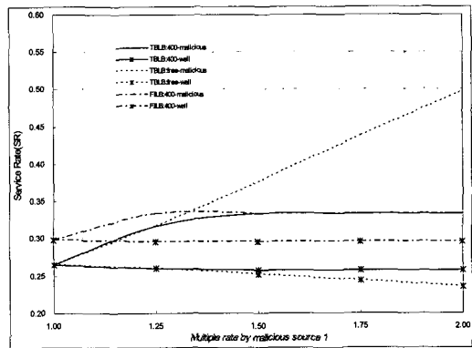
그림 4. 계약 위반 소스에 대한 각 연결의 서비스율
