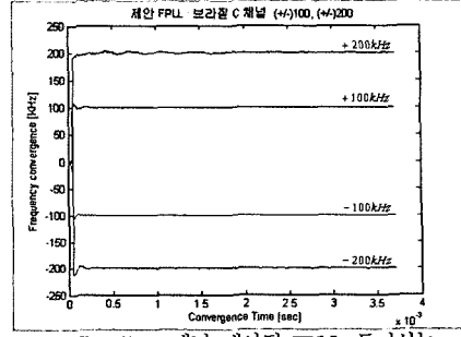
(b) Brazil C 채널 제안된 FPLL 동기성능
