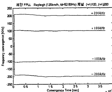
(b) Rayleigh(120km/h)에서 제안된 FPLL 동기 성능
