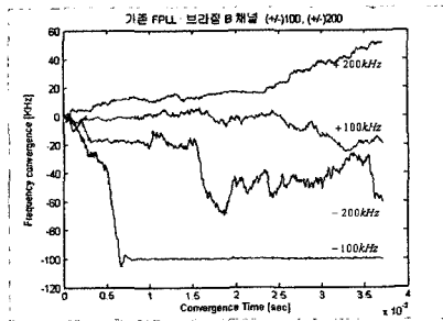
(a) Brazil B 채널에서 기존 FPLL 동기성능
