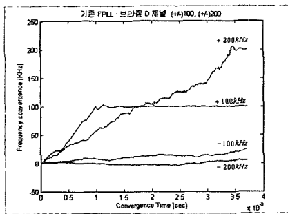
(a) Brazil D 채널에서 기존 FPLL 동기성능
