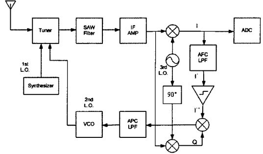
그림 2. 기존 FPLL의 블록도 Fig. 2. Block Diagram of the Conventional FPLL
