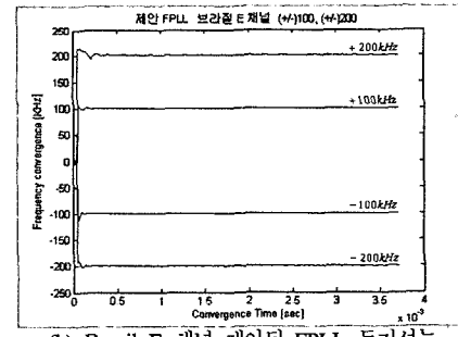
(b) Brazil E 채널 제안된 FPLL 동기성능
