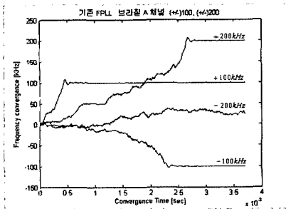
(a) Brazil A 채널에서 기존 FPLL 동기성능
