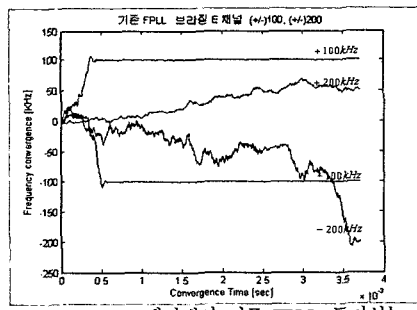
(a) Brazil E 채널에서 기존 FPLL 동기성능
