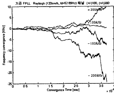
(a) Rayleigh(120km/h)에서 기존 FPLL 동기 성능
