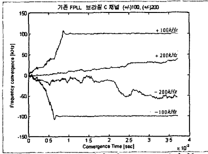
(a) Brazil C 채널에서 기존 FPLL 동기성능
