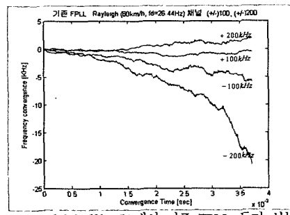
(a) Rayleigh(60km/h)에서 기존 FPLL 동기 성능
