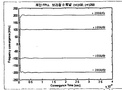
(b) Brazil D 채널 제안된 FPLL 동기성능
