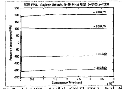
(b) Rayleigh(60km/h)에서 제안된 FPLL 동기 성능
