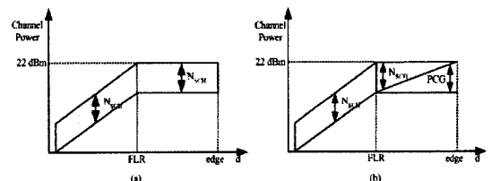
(a) PCG를 사용하지 않은 경우 (b) PCG를 사용한 경우 그림 4. OFDMA 시스템의 상향링크 송신전력
