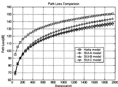
그림 5. 경로손실 모델비교
