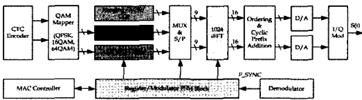
그림 1. HPI 시스템의 단말 송신기 구조
