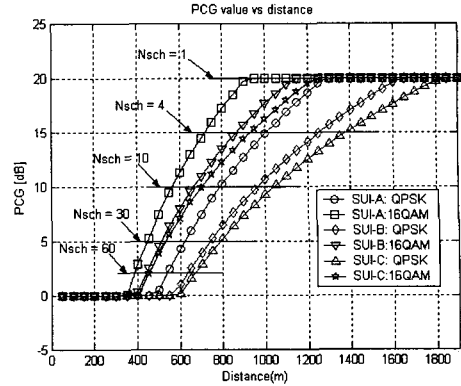
그림 7. N_{SCH} 에 따른 최대 통화반경
