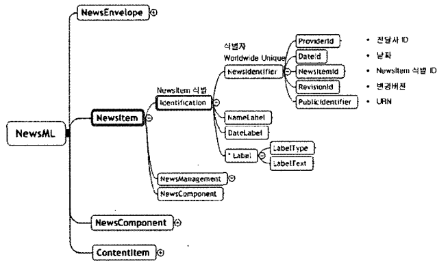
<그림 5> NewsML의 NewsItem 요소_1 (출처: 한국언론재단, 2004)
