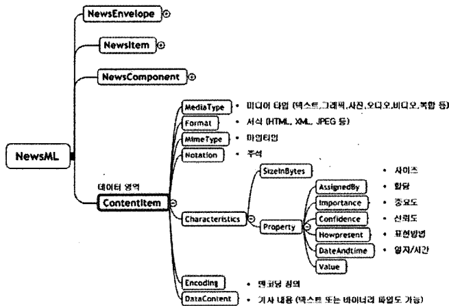
<그림 2> NewsML의 ContentItem 요소 (출처: 한국언론재단, 2004)
