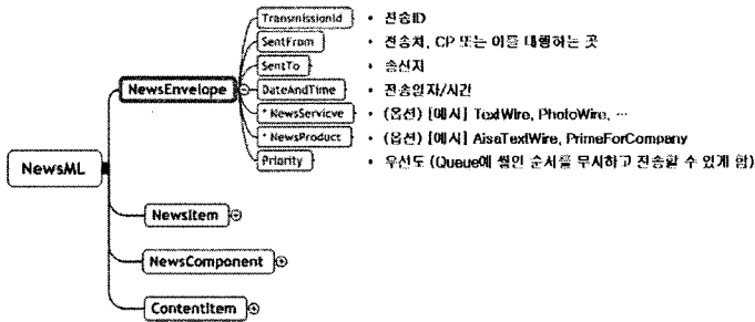
<그림 7> NewsML의 NewsEnvelope 요소 (출처: 한국언론재단, 2004)
