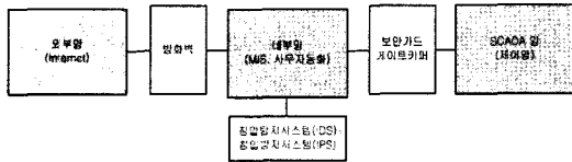
그림 6. SCADA 망에 대한 보안설계 구성도
