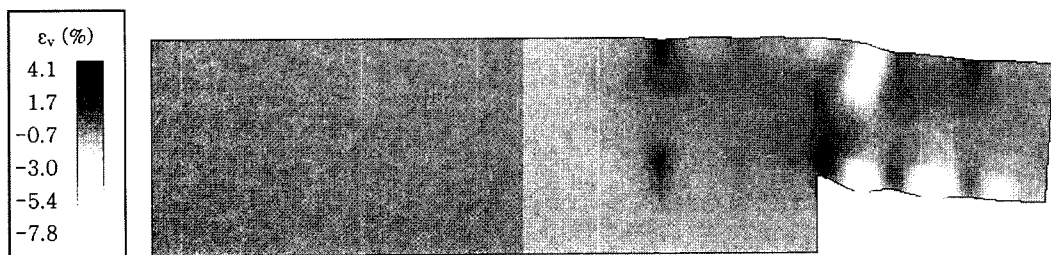
(c) 체적변형률 분포도
