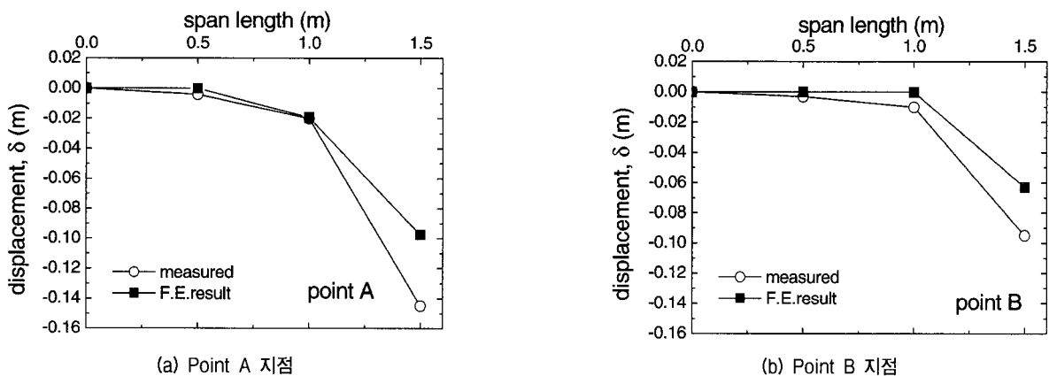
그림 16. 프리스트레스 하중을 고려하지 않은 각 계측점에서 성토 침하량 비교
