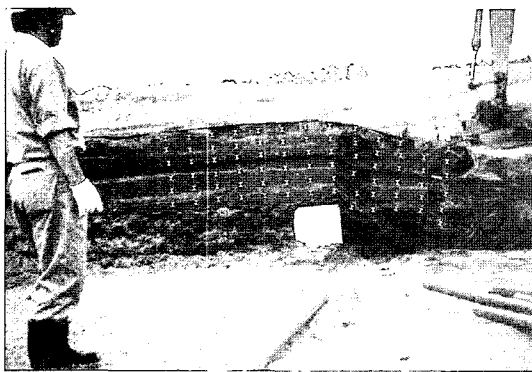
사진 3. 성토 A 변형(스판 길이 1.5m)
