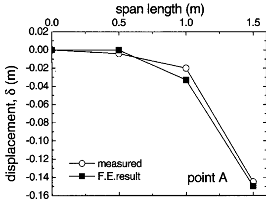
(a) Point A 지점
