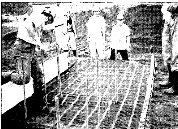
사진 1. 프리 스트레스 설치
