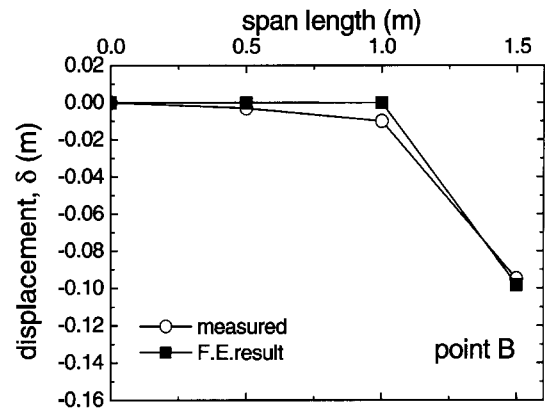
(b) Point B 지점
