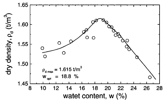
그림 5. 실내다짐시험 결과
