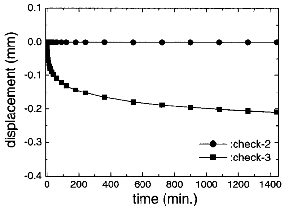
그림 10. 흙요소에 생긴 크리프 비교(check2, check3)
