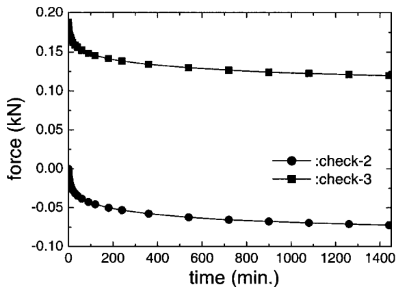
그림 11. 강봉이 받고 있는 프리스트레스 하중과 경과시간 변화
