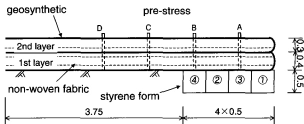
(a) 단면도(단위: m)
