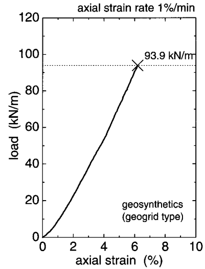
그림 4. 토목섬유의 인장시험 결과
