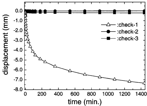
그림 9. 흙 요소에 생긴 크리프 비교
