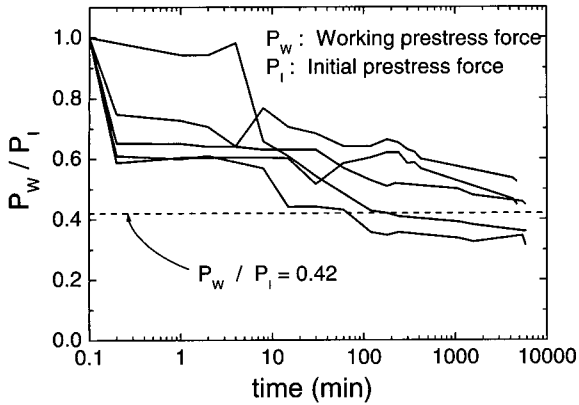
그림 17. 프리스트레스 유효 하중비와 시간변화의 관계
