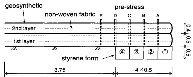
(a) 단면도(단위: m)
