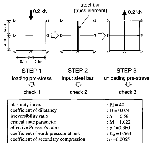
그림 8. 프리스트레스 모델화 검토
