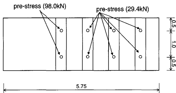
(b) 평면도(단위: m)
