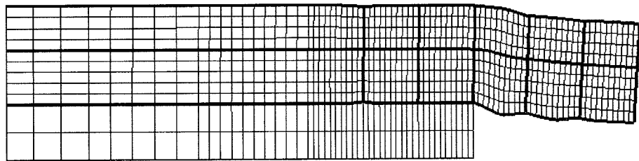
(a) 성토의 변형도
