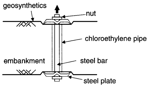
그림 3. 프리스트레스 설치 방법
