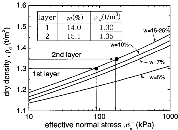
그림 14. 선행 압밀 응력 산정
