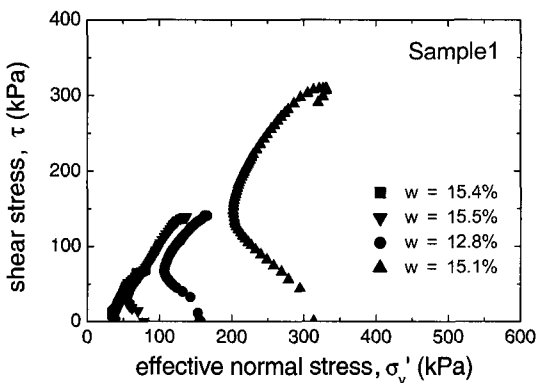
그림 6. 불교란 시료(다짐토)의 실내 시험 결과
