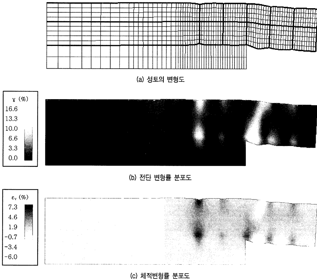
그림 15. 프리스트레스 하중을 고려하지 않은 유한요소 해석 결과
