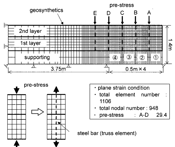
그림 12. 유한요소해석에 이용된 메쉬
