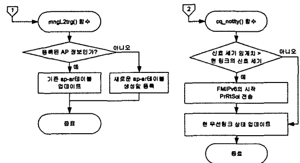
(그림 6) 제 2계층 트리거 발생 및 정보 갱신
