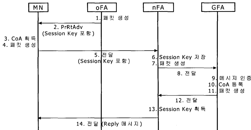
(그림 4) 기존의 세션키 재사용 핸드오프 방식
