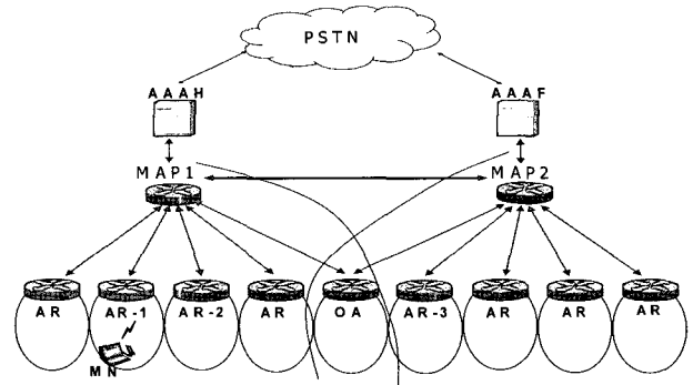
(그림 3) 제안하는 오버랩 네트워크 구조
