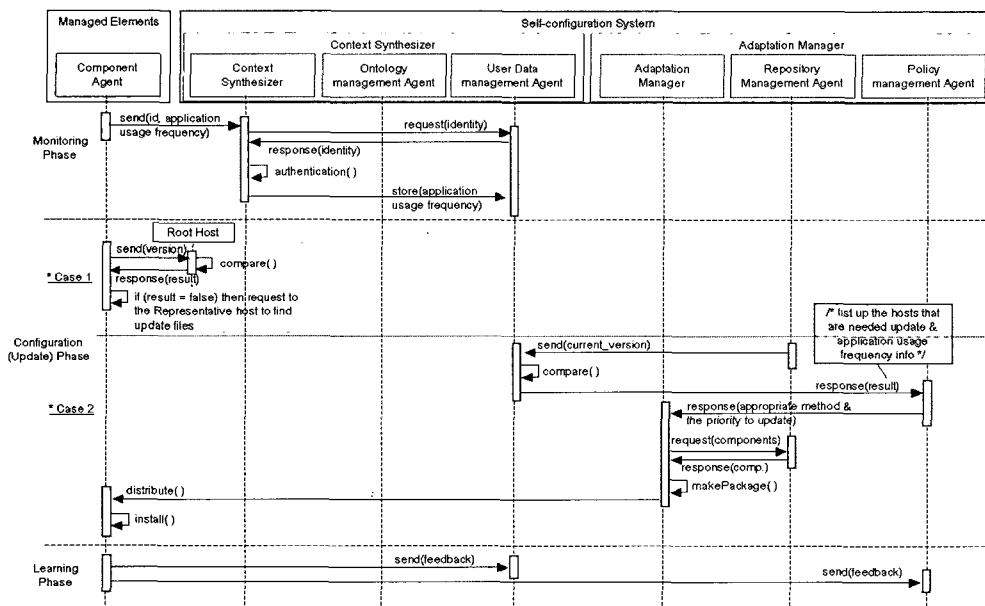
(그림 5) Update 과정의 시퀀스 다이어그램
