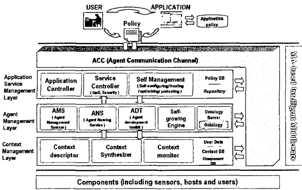
(그림 1) 멀티에이전트 기반 지능형 미들웨어의 구조
