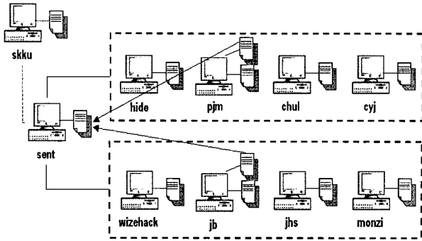
(그림 6) Peer-to-Peer전송을 위한 관리 대상들의 계층적 분류
