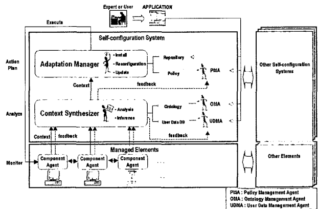
(그림 2) 제안 시스템의 전체적인 구조
