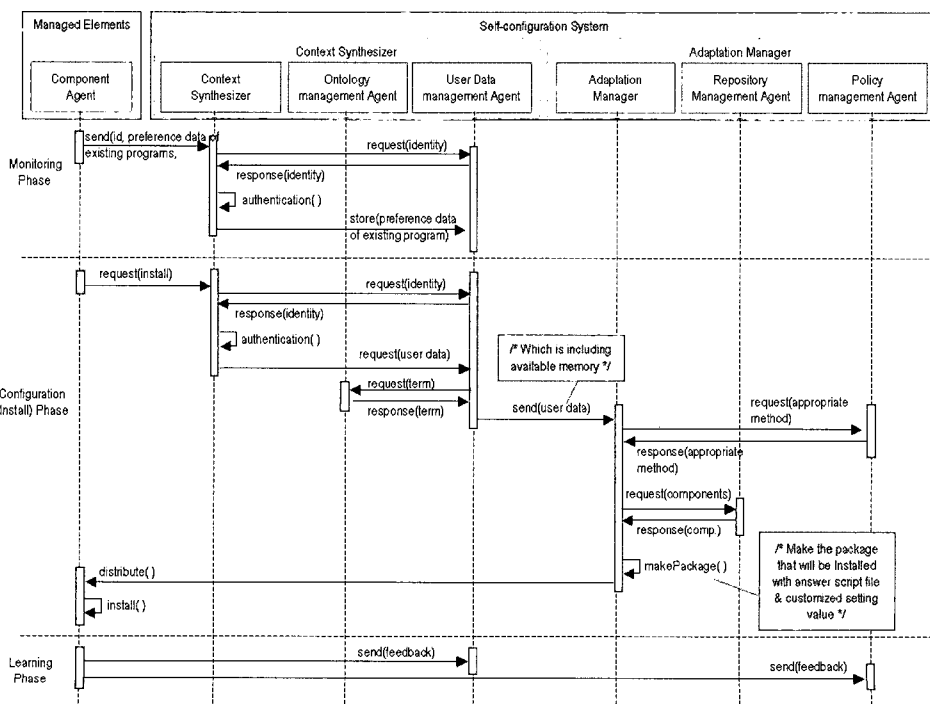
(그림 3) Install 과정의 시퀀스 다이어그램
