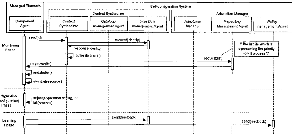
(그림 4) Reconfiguration 과정의 시퀀스 다이어그램
