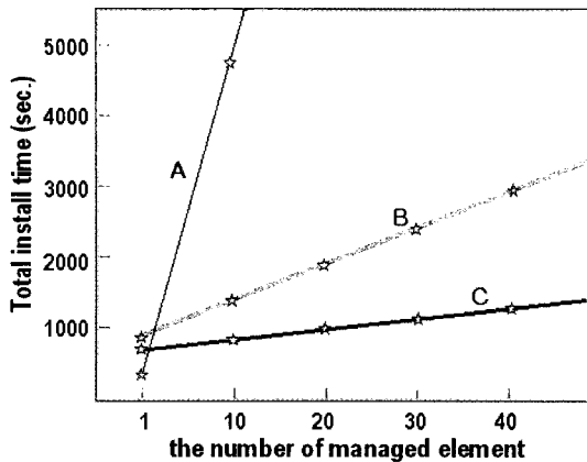
(그림 10) 세 방식의 Install time 비교 그래프
