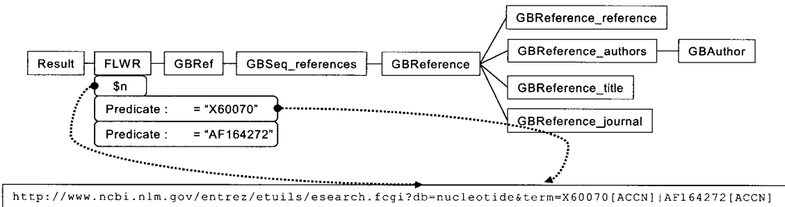
(그림 14) 합성된 질의 트리로부터 URL 형식으로 변환하는 과정
