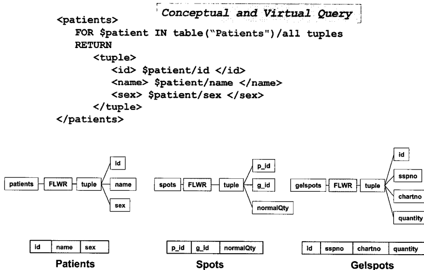
(그림 5) 가상적인 XQuery와 대응되는 기본 XML 뷰 트리
