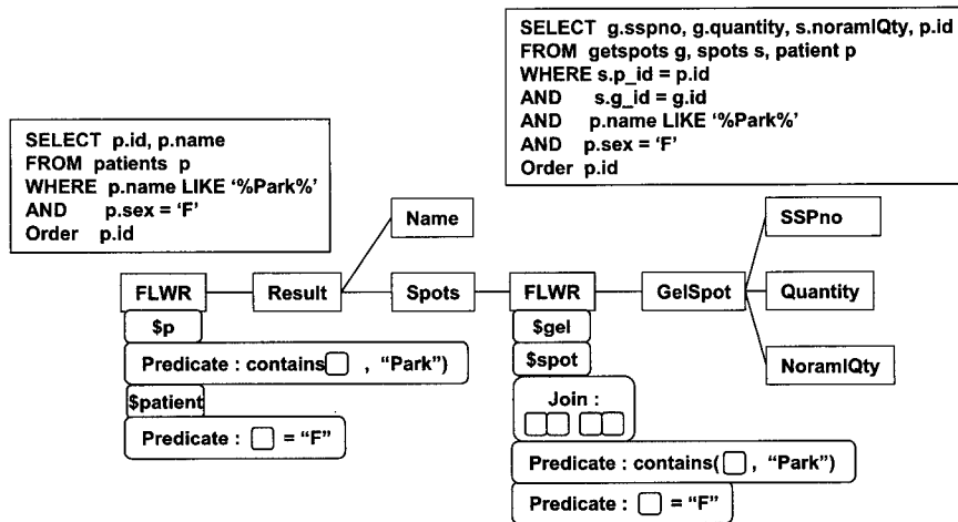
(그림 12) 디코릴레이션된 질의 트리화 생성된 SQL
