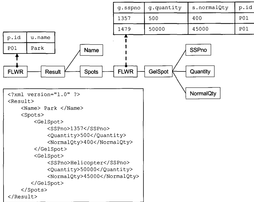
(그림 15) SQL 수행 결과와 변환된 XML 문서
