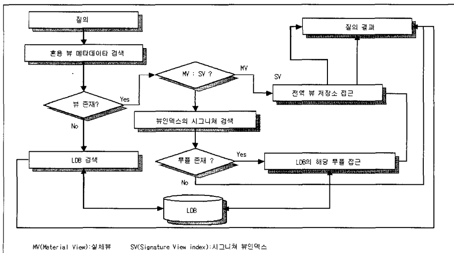
(그림 4) 뷰 관리 혼용 기법
