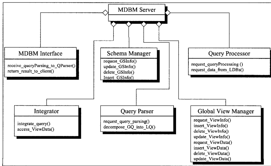
(그림 7) MDBM 서버의 클래스 다이어그램
