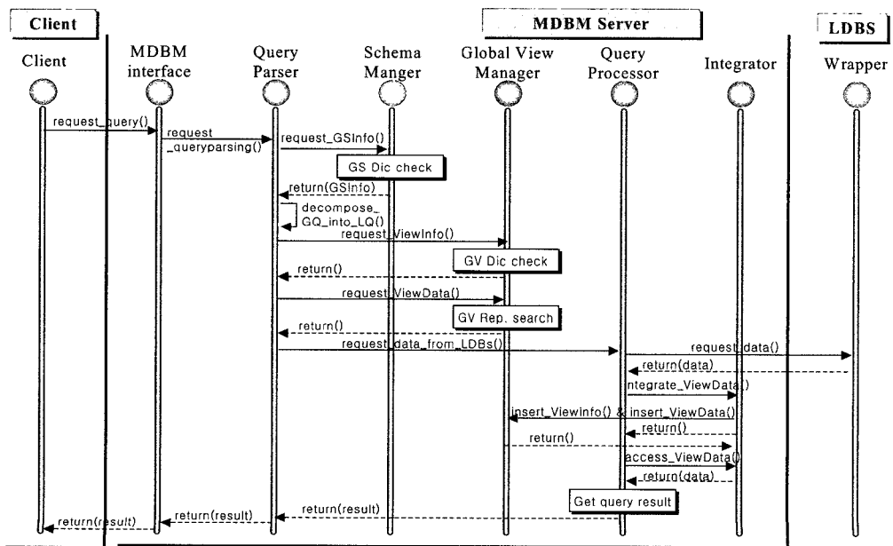
(그림 12) Nothing인 경우의 시퀀스 다이어그램
