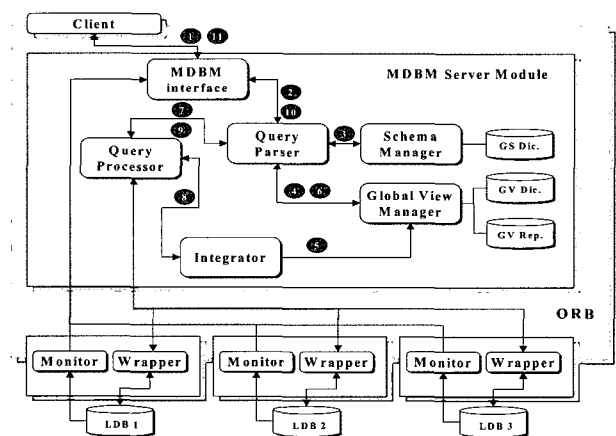
(그림 8) ALL : 모든 부분 질의에 대한 뷰가 존재
