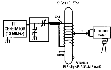
그림 3. 실험 장치 계략도.
