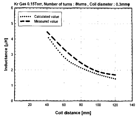
그림 9. 코일의 간격 변화에 따른 인덕턴스 특성. Fig. 9. Inductance dependence on coil distance.
