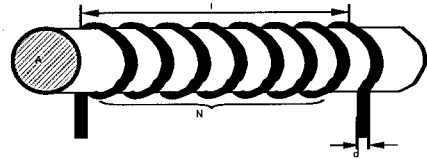
그림 1. 유도결합형 플라즈마 방전관.
