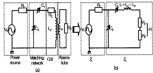
그림 2. 유도결합형 플라즈마 방전관의 전기적인 등가 회로.
