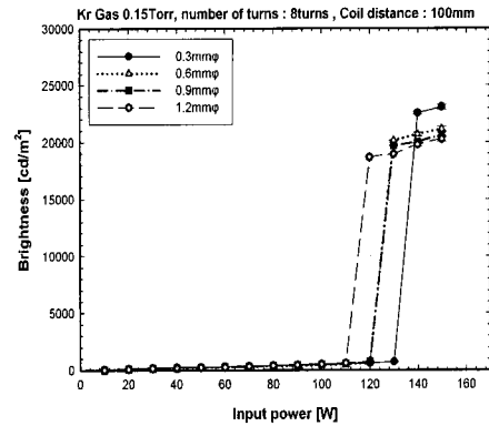
그림 5. 코일의 직경과 RF 전력변화에 따른 휘도 특성.
