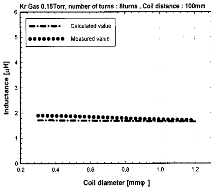
그림 4. 코일의 직경 변화에 따른 인덕턴스 특성. Fig. 4. Inductance dependence on coil diameter.
