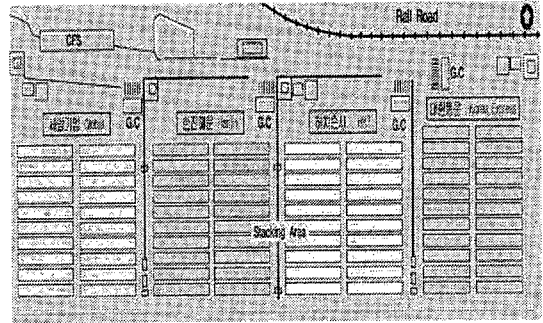
그림 4. 감만 컨테이너부두 터미널 배치도
