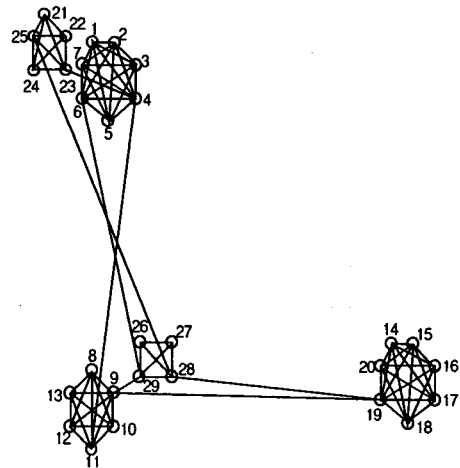
그림 9. 계층적 라우팅을 위한 그래프 모델(2계층의 확장 그래프) Fig 9. A graph model for a hierarchical routing (the extended graph of 2 layer)
