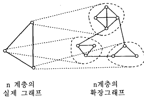
그림 1. 확장그래프 예제 Fig 1. An example of the extended Graph
