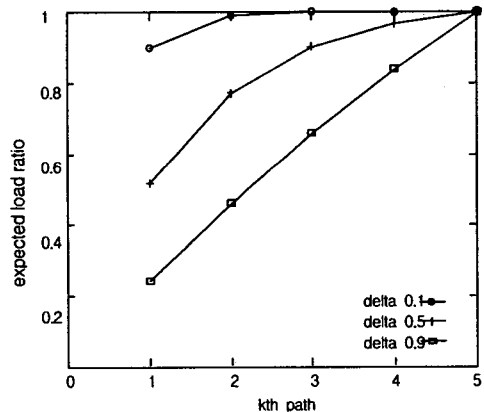
그림 5. K=5에서의 예측부하율( L_k(e) ) Fig 5. The expected load ratio in K=5
