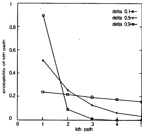
그림 6. K=5 에서의 k^{th} 경로들의 경로선택 확률 Fig 6. The probability of the k^{th} path selection in K=5
