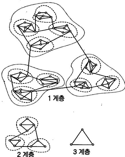
그림 2. 계층적 도메인 예제 Fig 2. A example of the hierarchical domain
