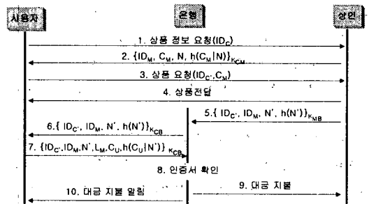
그림 5 지불 프로토콜 Fig 5. Payment protocol
