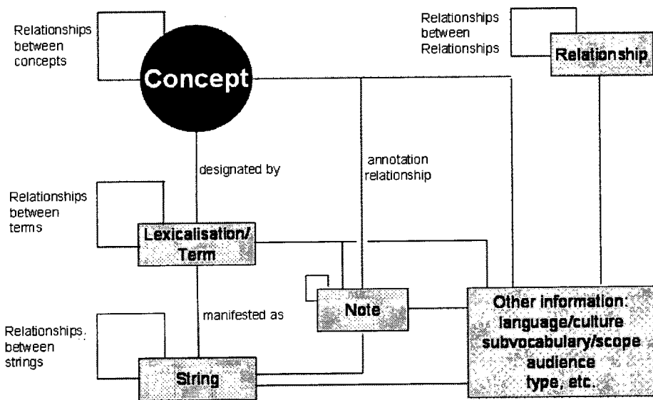
<그림 3> 시소러스와 온톨로지의 통합을 위한 개념 모형
