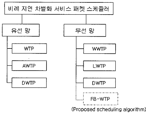
그림 1. 비례 지연차별화 서비스 스케줄링 알고리즘
