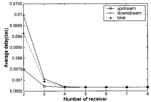
그림 6. Receiver 수의 증가에 따른 평균지연시간 (RTT=0)
