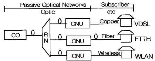
그림 1. PON의 구조 및 확장성
