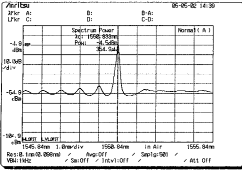
(a) CO에서 RN까지의 스펙트럼
