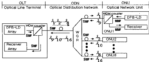
그림 2. 전송 시스템 구조
