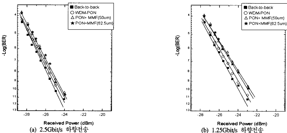
그림 6. 하향전송 BER 곡선
