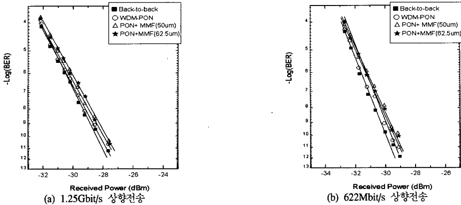
그림 7. 상향 전송 BER 곡선
