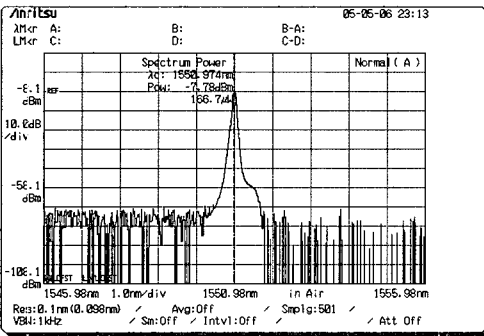
(b) ONU에서의 스펙트럼
