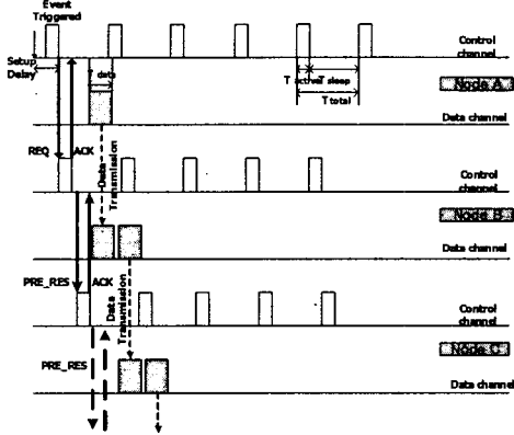
그림 3. 작은 크기의 패킷 전송시 LEEM의 문제점 Fig 3. Problem of LEEM by small size Packet
