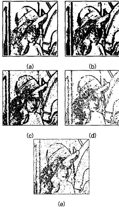
그림 4. (a)는 Wilcoxon 검정, (b) T 검정, (c) Sobel 방법, (d) Canny 방법, (e) Wavelet 변환방법을 그림 2(b)에 적용하여 얻은 에지맵이다. Fig 4. Edge detection results for Lenna image in Fig 2(b): (a) Wilcoxon test (b) T test (c) Sobel detector (d) Canny detector (e) Wavelet detector
