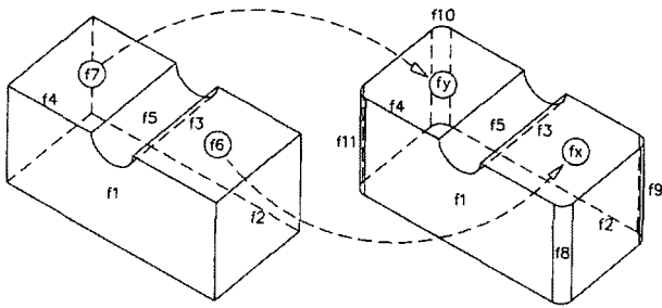
Fig. 5-1. Local matching (Problem 2).
