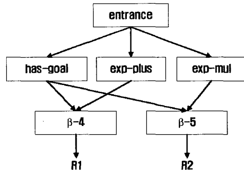
그림 2. Rete 네트 구조
