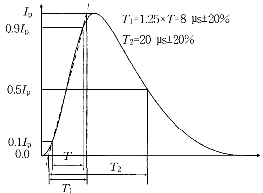
그림 2. 전형적인 썬지전류 파형.
