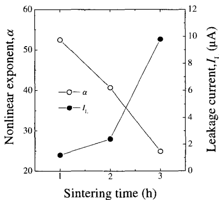
그림 6. 소결시간에 따른 바리스터의 비직선 지수와 누설전류.
