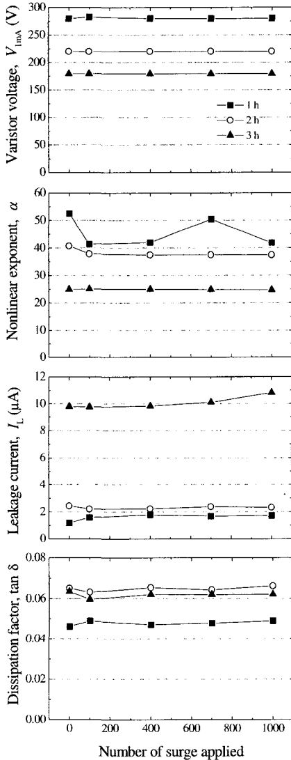
그림 8. 바리스터의 소결시간별 써지 스트레스 전·후의 전기적 특성 파라미터 변화.
