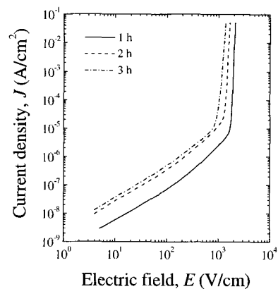
그림 4. 소결시간에 따른 바리스터의 E-J 특성.
