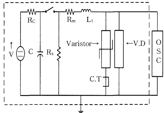
그림 1. 썬지시험장치의 개략도.
