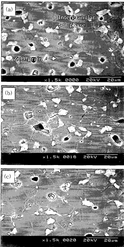
그림 3. 바리스터의 소결시간별 SEM 사진; (a) 1시간, (b) 2시간, (c) 3시간.
