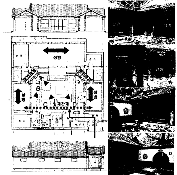
<그림 10>가족관계에 따른 사합원(在四八秀其吳四合院) 도면 및 사진 출처: 馬炳堅(1999), 北京四合院建築, 天津大學出版社.
