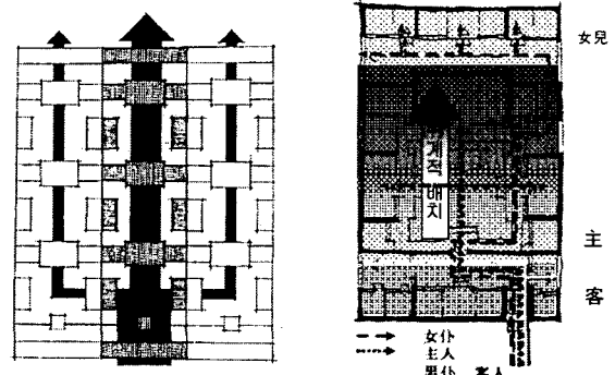
사합원의 공간분화원리 사합원의 배치원리 출처: 王其明 外 1人(1996), 北京四合院, 中國建築工業出版社
