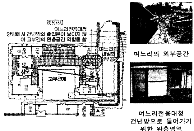
<그림 7>고부관계에 따른 안채의 공간표현(윤증고택) 도면출처: 「한옥의 향기」, 대원사
