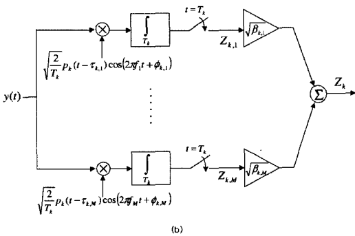
그림 1. 본 논문에서 고려하는 MC-CDMA 방식의 송수신기의 구조도 (a) 송신부 (b) 수신부
