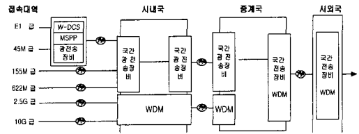
그림 6. 전달망의 대역별 접속설비기준 모델
