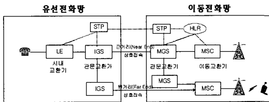
그림 1. 유선전화와 이동전화간의 상호접속
