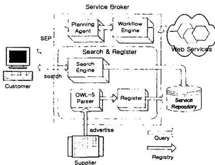
그림 10. IMP 시스템 구조 Fig. 10. IMP system architecture
