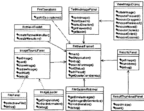
그림 9. 키워드와 예제 이미지의 통합을 이용한 검색 클래스 다이어그램
