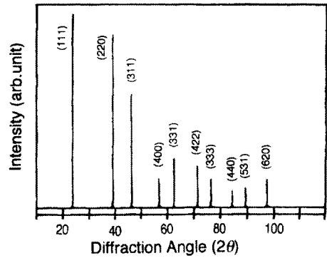
그림 3. 분말법에 의한 x-선 회절 peak Fig. 3. X-ray diffraction peak for powder method.
