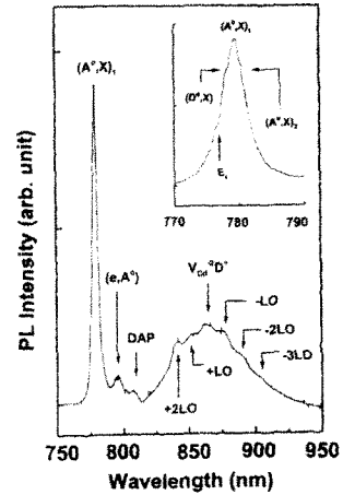
그림 6. 10 K에서의 광발광 스펙트럼 Fig. 6. Photoluminescence spectrum at 10 K.
