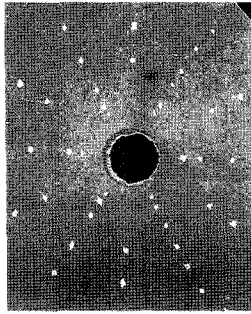
그림 4. Laue 배면반사법에 의한 (111)면의 Laue pattern Fig. 4. Laue pattern of (111) plane for Laue back reflection.
