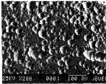
그림 5. SEM에 의한 (111)A면의 전형적인 etch pits 표면 형상 사진 Fig. 5. Typical etch pits surface picture of (111)A plane for SEM.
