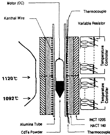
그림 1. 수직 Bridgman 방법의 전기로 및 온도구배 Fig. 1. Furnance and temperature gradient for vertical Bridgman method.
