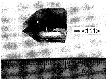
그림 2. 수직 Bridgman 방법으로 성장된 CdTe 단결정 사진 Fig. 2. Photographic of CdTe single crystal grown by vertical Bridgman method.
