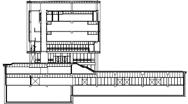
종단면도
