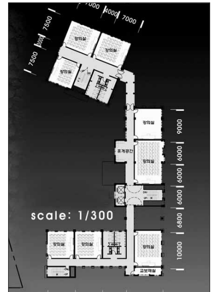
2층 평면도
