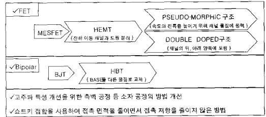
(그림 3) 고주파 반도체소자의 새로운 구조에 의한 성능 향상
