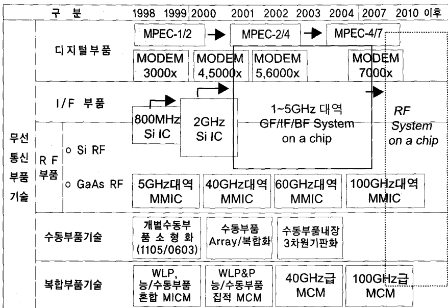
(그림 9) 주요부품의 기술전망
