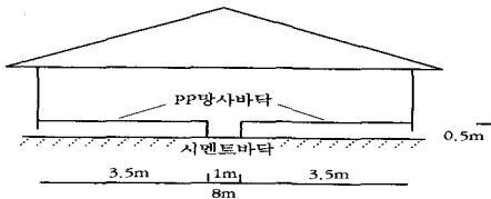
<그림1> 일반적인 육계사
