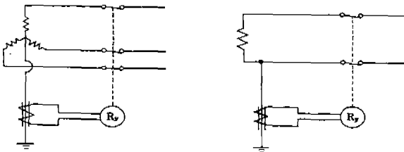
그림 4 누전차단방식의 예
