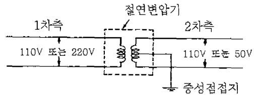
(b)중성점접지식 전로
