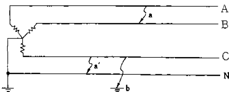
그림 1 단락과 지락
