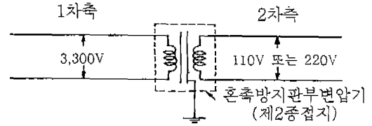
(a)비접지식 전로
