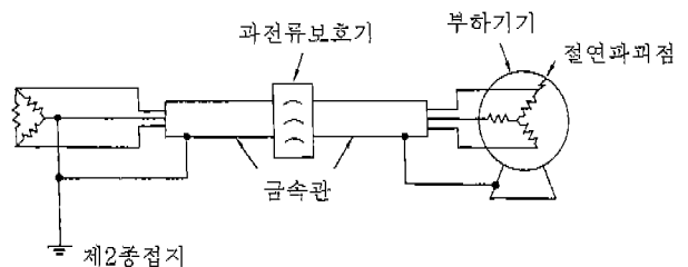
그림 3 과전류차단방식의 예
