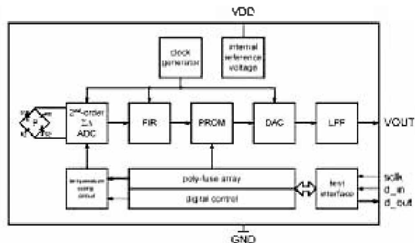
그림8. Smart Pressure Sensor
