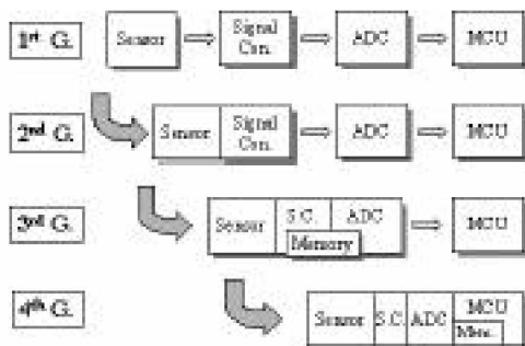
그림 2. 스마트 센서의 개념 및 발전과정
