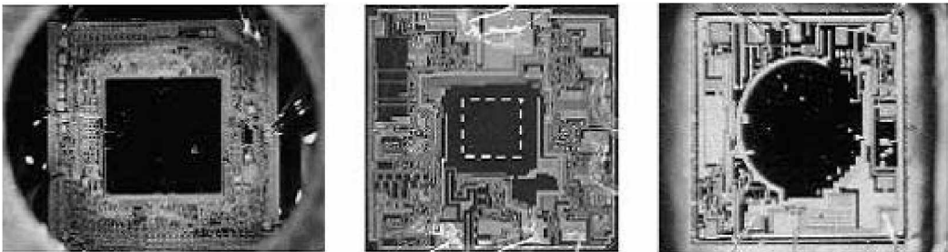
그림7. Integrated Pressure Sensor
