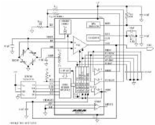
그림6. digital trimming을 적용한 압력센서용 스마트 IC
