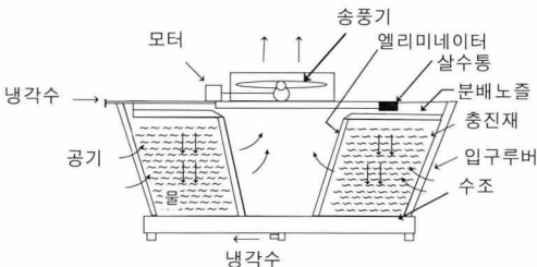
〈그림 2〉 직교류형 냉각탑
