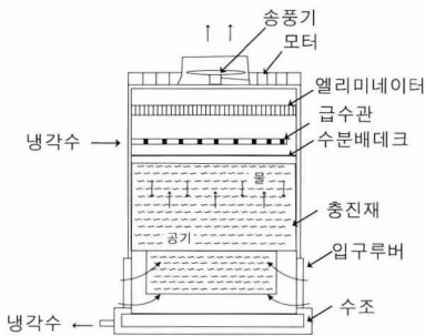
〈그림 1〉 향류형 냉각탑
