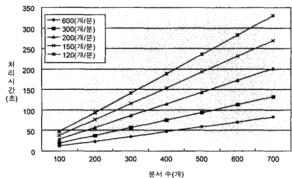
(그림 6) 데이터 유입률에 따른 문서 처리시간
