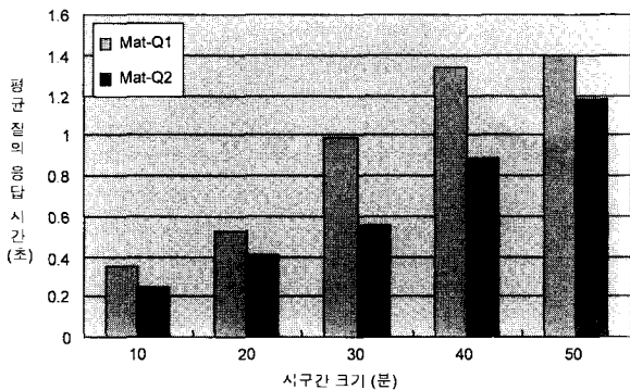
(그림 9) 시구간 크기에 따른 질의 응답시간
