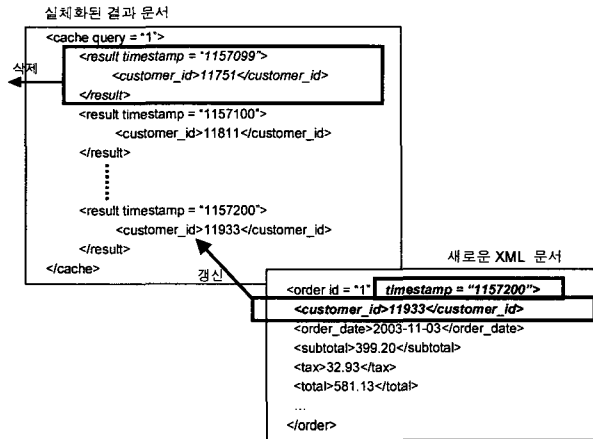
(그림 4) 질의 결과의 점진적 갱신
