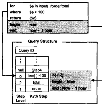
(그림 2) QS 자료구조
