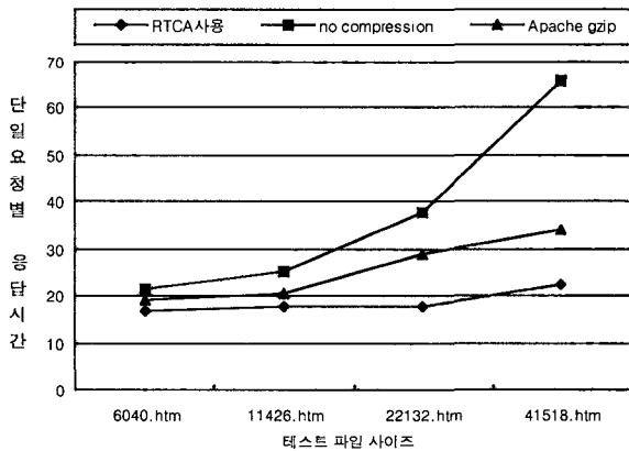
(그림 4) 테스트 파일 사이즈별 서버측의 단일요청별 응답시간
