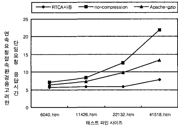
(그림 5) 테스트 파일 사이즈별 연속요청 접속 환경을 고려한 단일요청별 응답 시간
