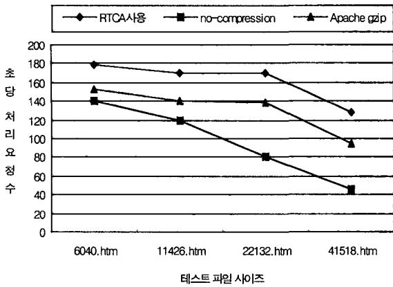
(그림 3) 테스트 파일 사이즈별 서버측의 초당 처리 요청수
