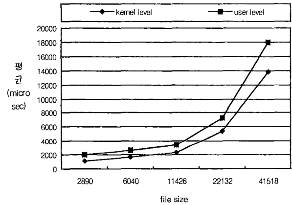
(그림 1) 사용자/커널 영역에서의 압축수행시간 비교
