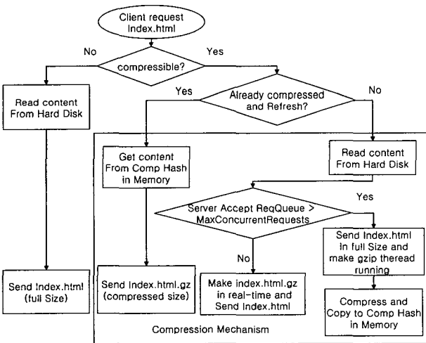
(그림 2) 실시간 압축전송 알고리즘도
