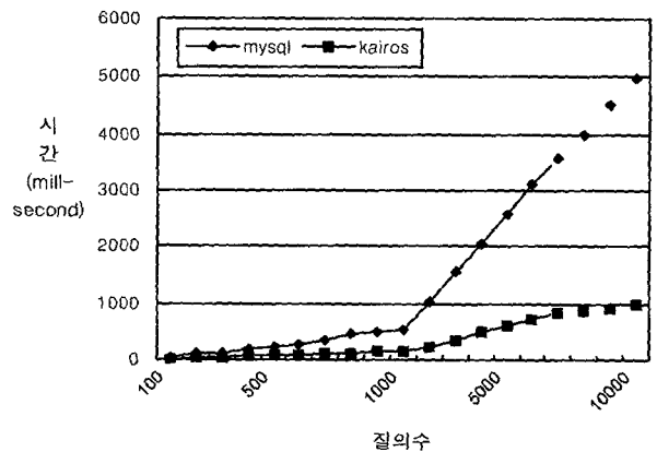
(그림 7) ldap_search 비교 그래프
