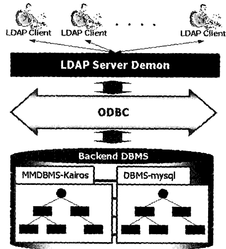
(그림 6) 실험환경
