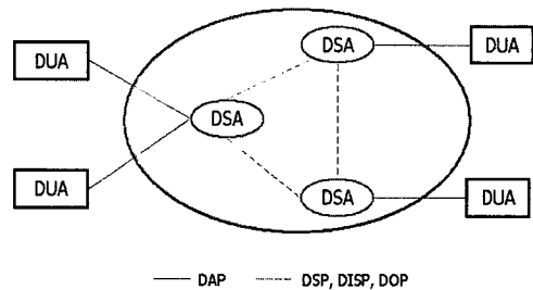
(그림 2) X.500 디렉토리 서비스 시스템
