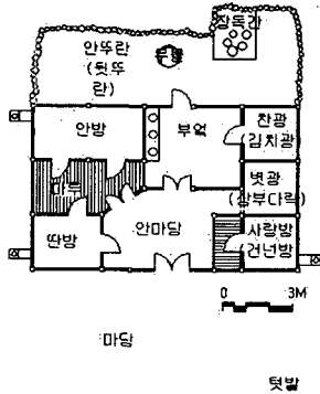
그림 5. 교동면 고구리 황경준씨 집
