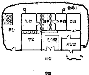
그림 23. 한채로 지어 경제적인 트입구집 (북쪽측)
