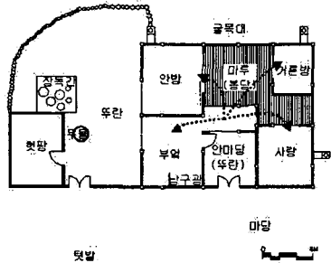
그림 19. 동선의 내부공간화 (서덕용씨 집 고친 후)
