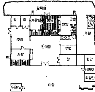
그림 24. 상류주거로서의 튼입구집 (신상영)
