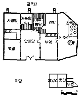
그림 4. 특입구자집. 하점면 창후리 김순동씨 집
