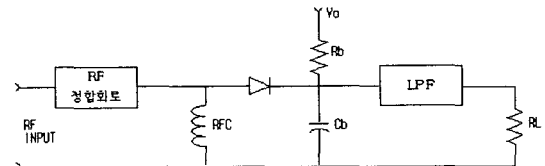
그림 2. 다이오드 검파기 회로 Fig 2. Diode detector circuit.
