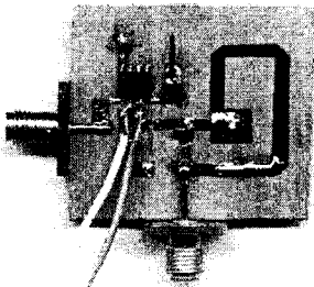
그림 5. 제작된 다이오드 검파기 Fig 5. Fabricated diode detector.
