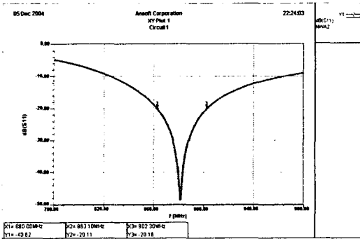
그림 8. 로그 칩형 검파기의 시뮬레이션 결과 Fig 8. Simulation result of log chip detector.
