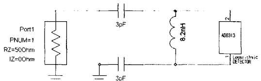
그림 7. 로그 칩형 검파기의 입력 정합회로 Fig 7. Input matching circuit of log chip detector.
