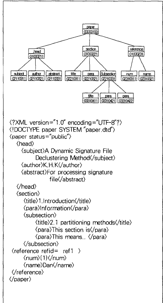
그림 1 트리아구조를 이용한 XML 문서의 구조 Fig. 1 XML document information representation using Tree structure
